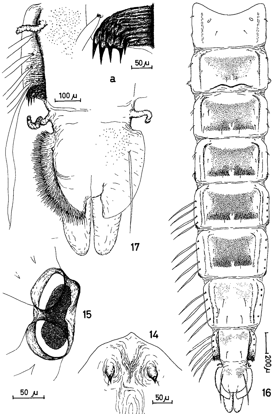
Tafel VI: Siolimya amazonica , Puppe
