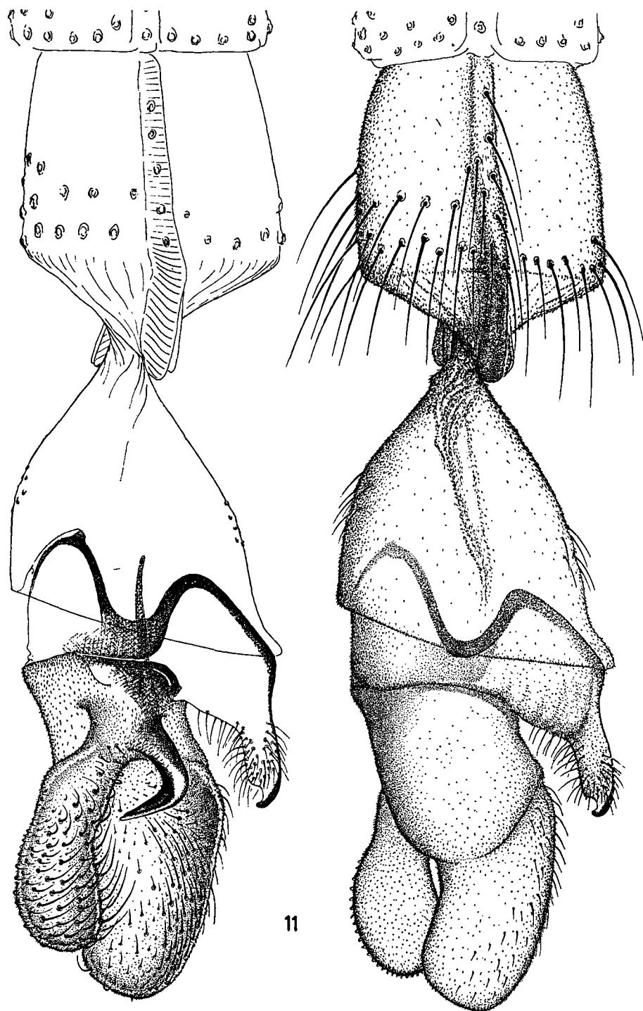
Tafel IV: Siolimya amazonica , Imago ♂
