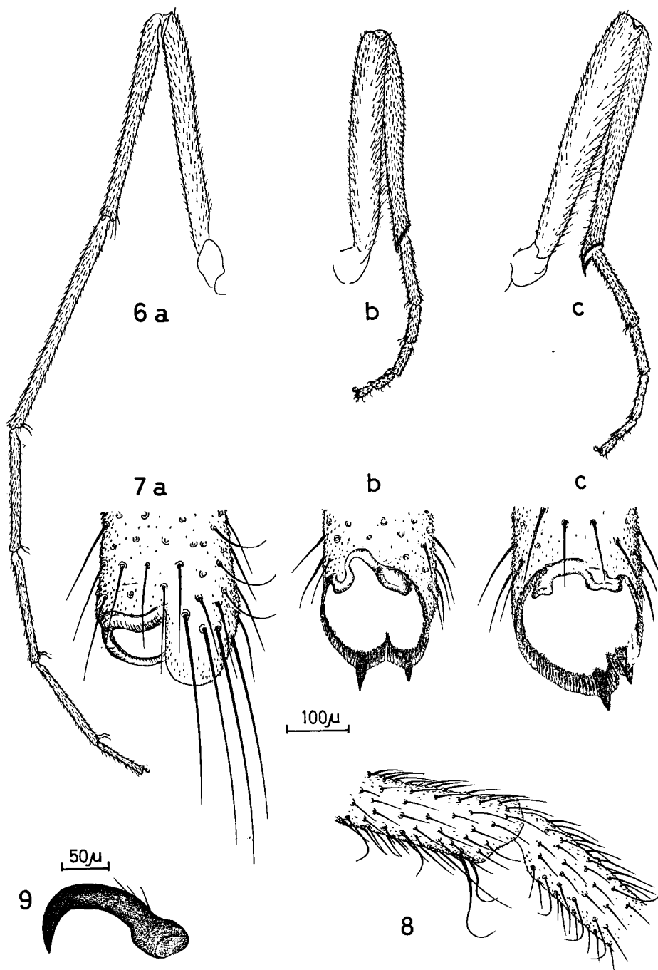
Tafel II: Siolimya amazonica , Imago ♂
