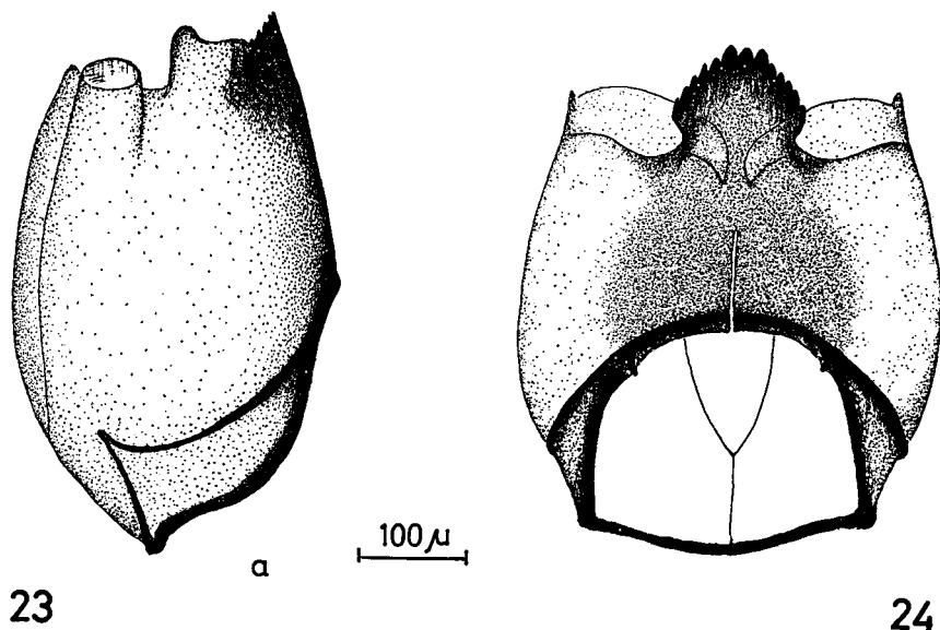
Tafel VIII: Siolimya amazonica , Larve
