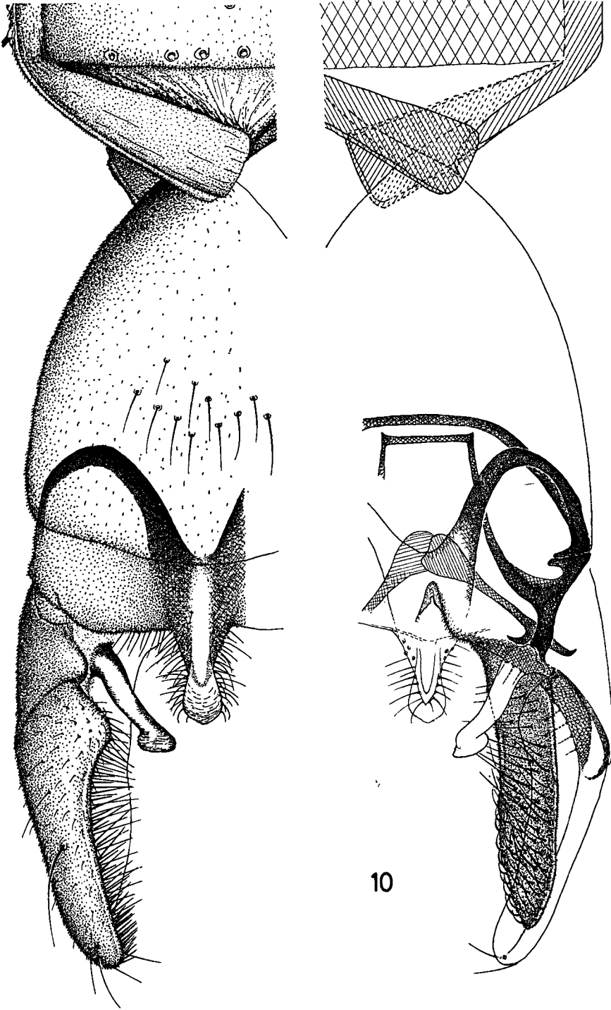
Tafel III: Siolimya amazonica , Imago ♂
