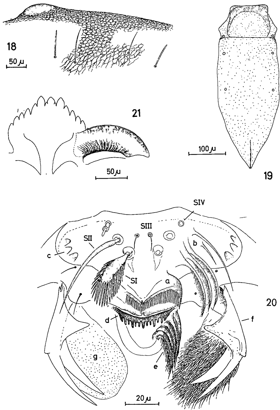
Tafel VII: Siolimya amazonica , Puppe, Larve
