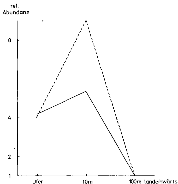
Abb. 2: Relative Abundanz der Carabidae (— — — —) und aller Käfer (—) im Überschwemmungswald bei steigender Flut. Die Zahl der Käfer je Probe bei 100 m im Landesinnern wurde gleich 1 gesetzt.
