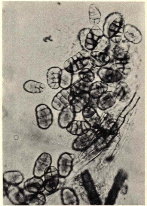
Abb. 21 : Darmausstriche von Asseln. Die wesentlichen noch erkennbaren Nahrungsbestandteile sind Hyphenstücke und Sporen von Pilzen (Hochwald, Reserva Ducke bei Manaus).
