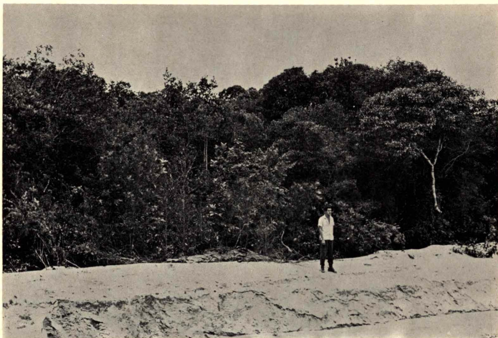
Abb. 10 : Caatinga baixa (Km 208 an der Straße Manaus — Itacoatiara).
