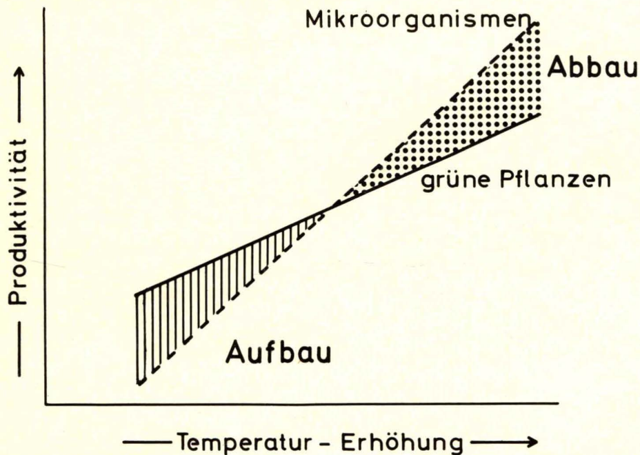
Abb. 24 : Schema des Einflusses der Temperatur auf Wachstum und Vermehrung der grünen Pflanzen (Produzenten) und Mikroorganismen (Reduzenten) und den Aufbau und Abbau von Humus am Boden.
