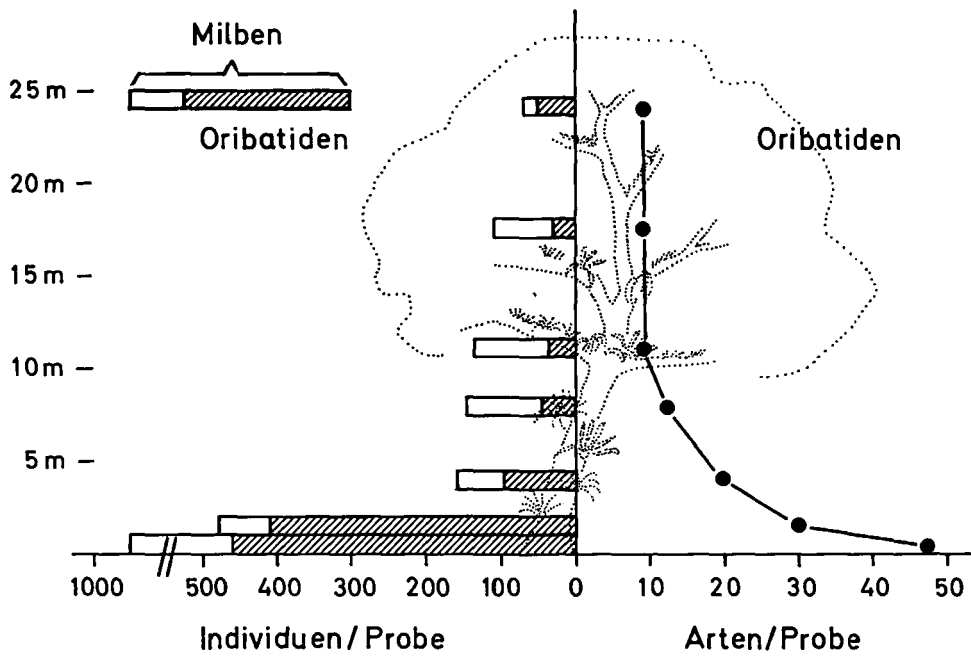
Abb. 19 : Individuen- und Arten-Abundanz der Milben und Oribatiden des „Epiphytenhumus“ in verschiedener Höhe über dem Boden (Caatinga, Reserva Ducke bei Manaus; vergl. Abb. 11).
